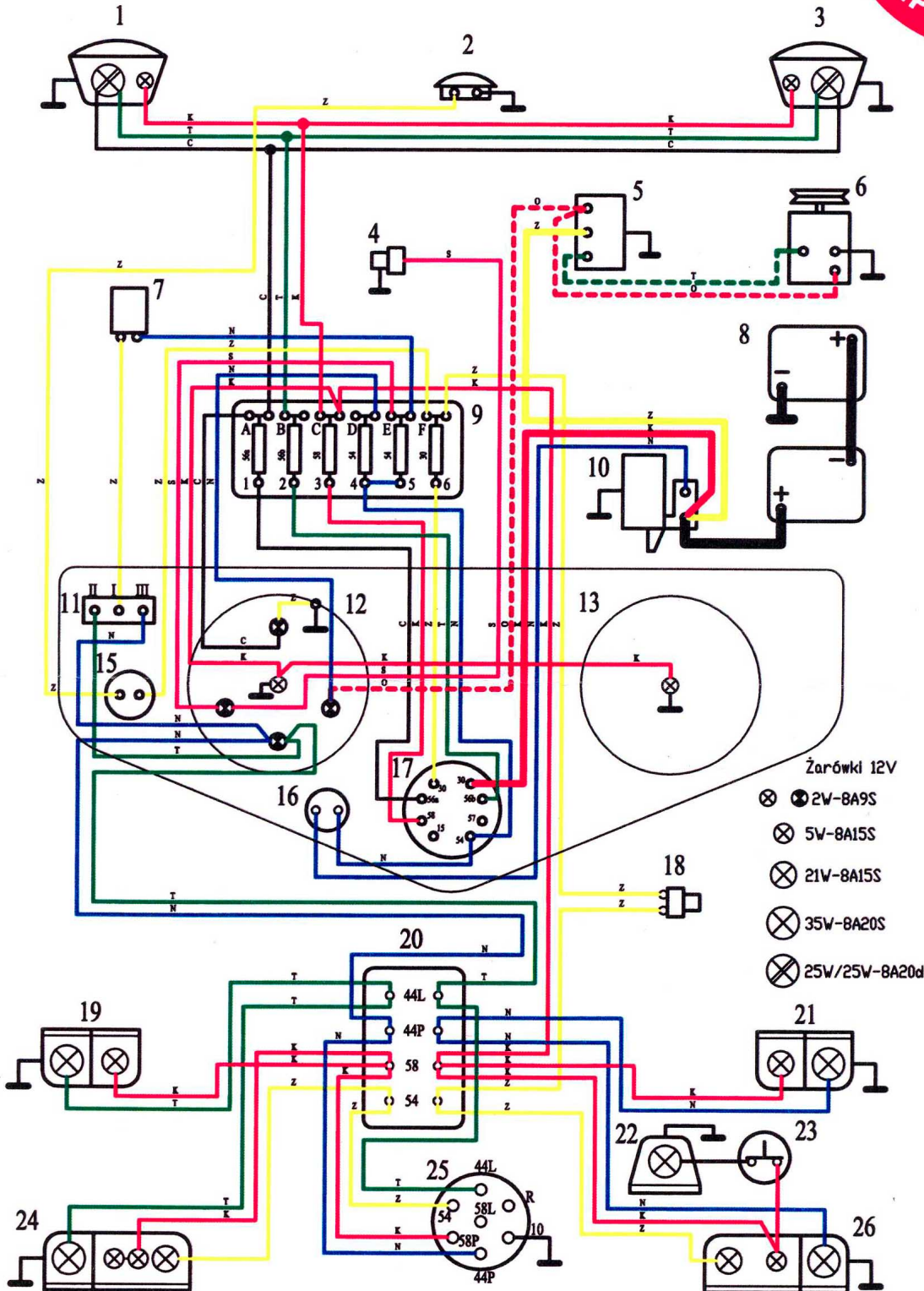
Schemat instalacji elektrycznej C-360 (prądnica)
